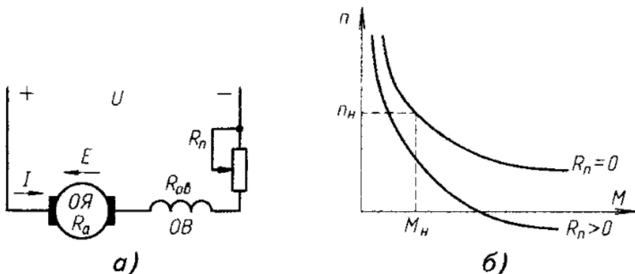
Рисунок 5 – Система включения (а) и механические характеристики (б) двигателя постоянного тока параллельного возбуждения
