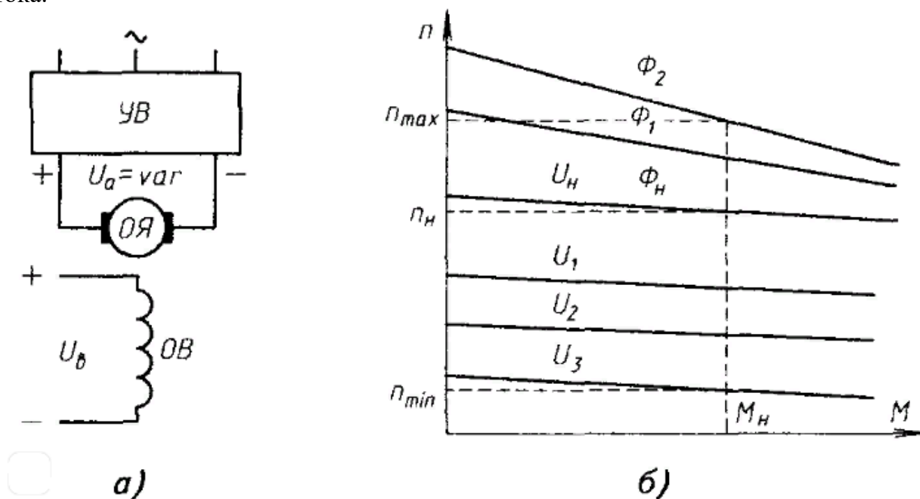
Рисунок 4 – Система «управляемый выпрямитель – двигатель» (а) и механические характеристики при изменении напряжения на якоре и магнитного потока (б)
