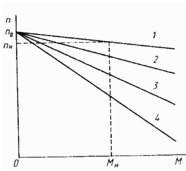
Рисунок 3 – Механические характеристики двигателя постоянного тока параллельного возбуждения
