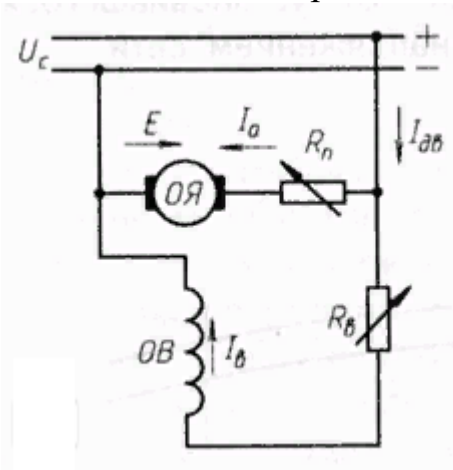
Рисунок 2 – Схема включения двигателя постоянного тока параллельного возбуждения в сеть
